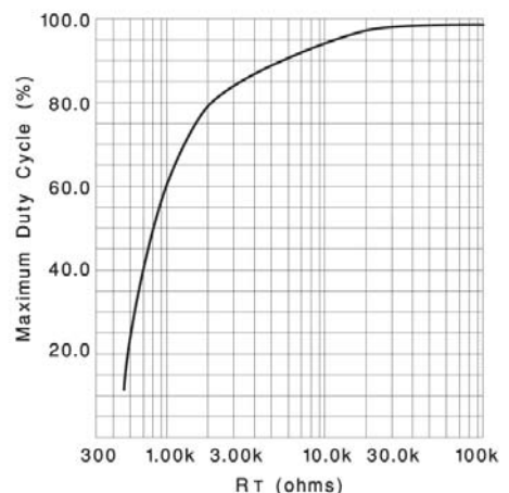
最大占空比
