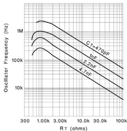
频率与电阻
