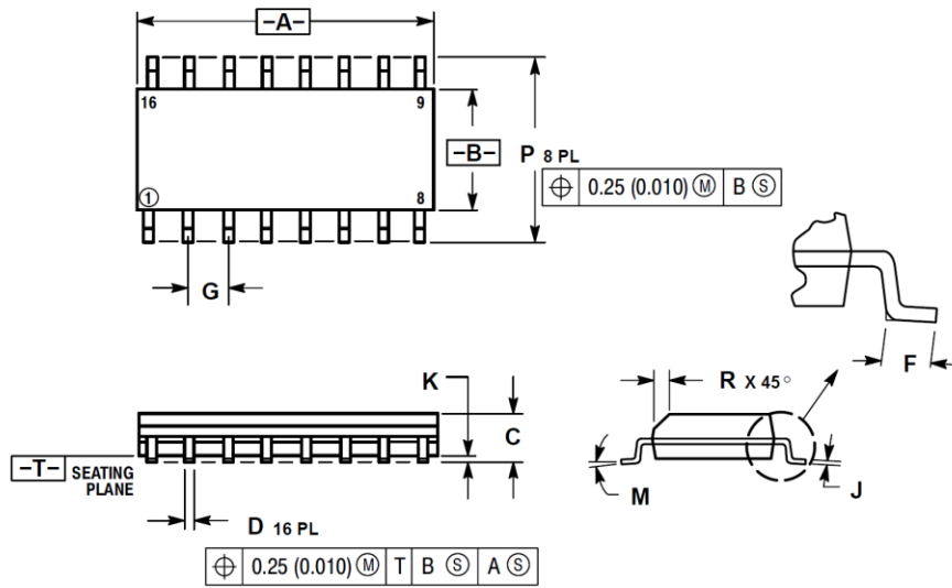
SOP16
